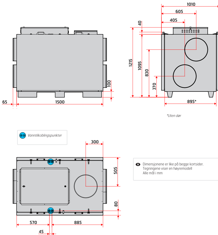
Målskisse L20 R
